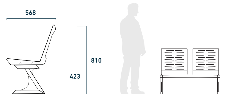
Vista Lateral
